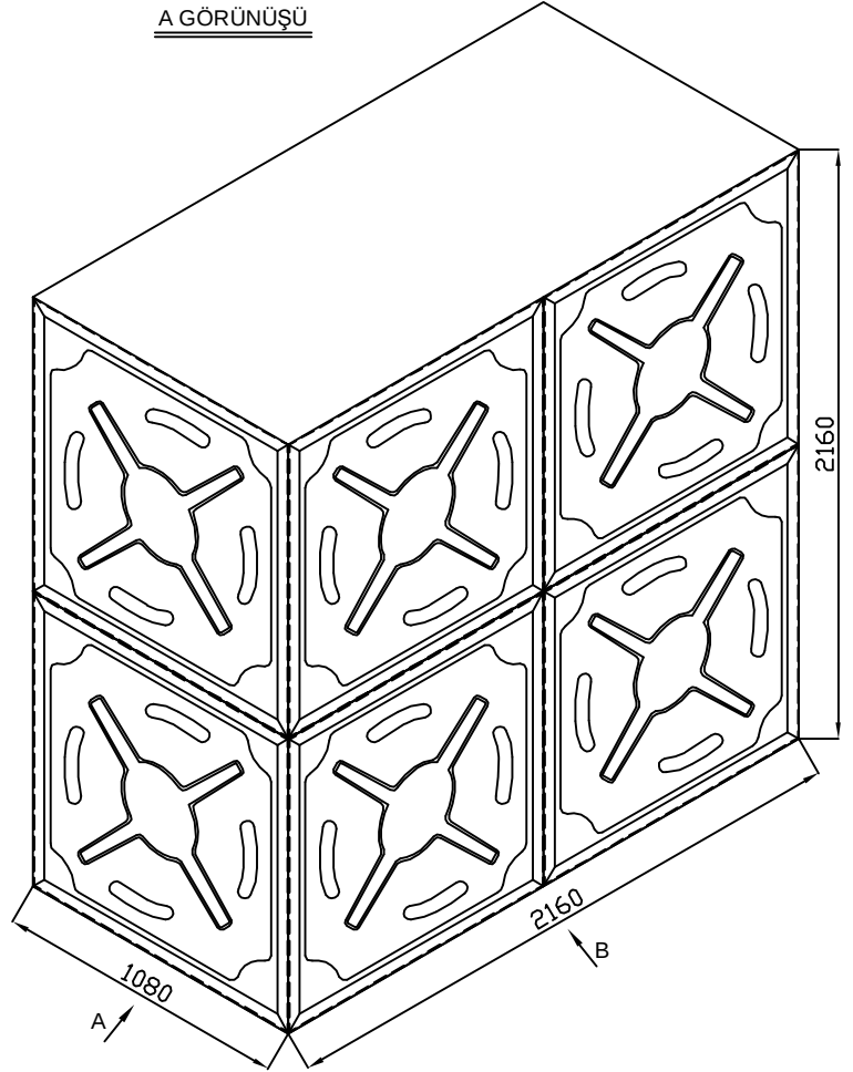
GENEL GÖRÜNÜŞ
