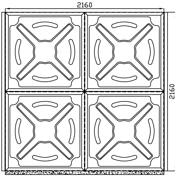
B GÖRÜNÜŞÜ
