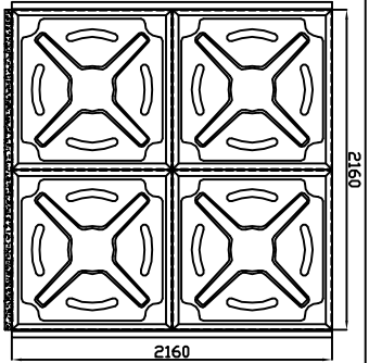
A GÖRÜNÜŞÜ
