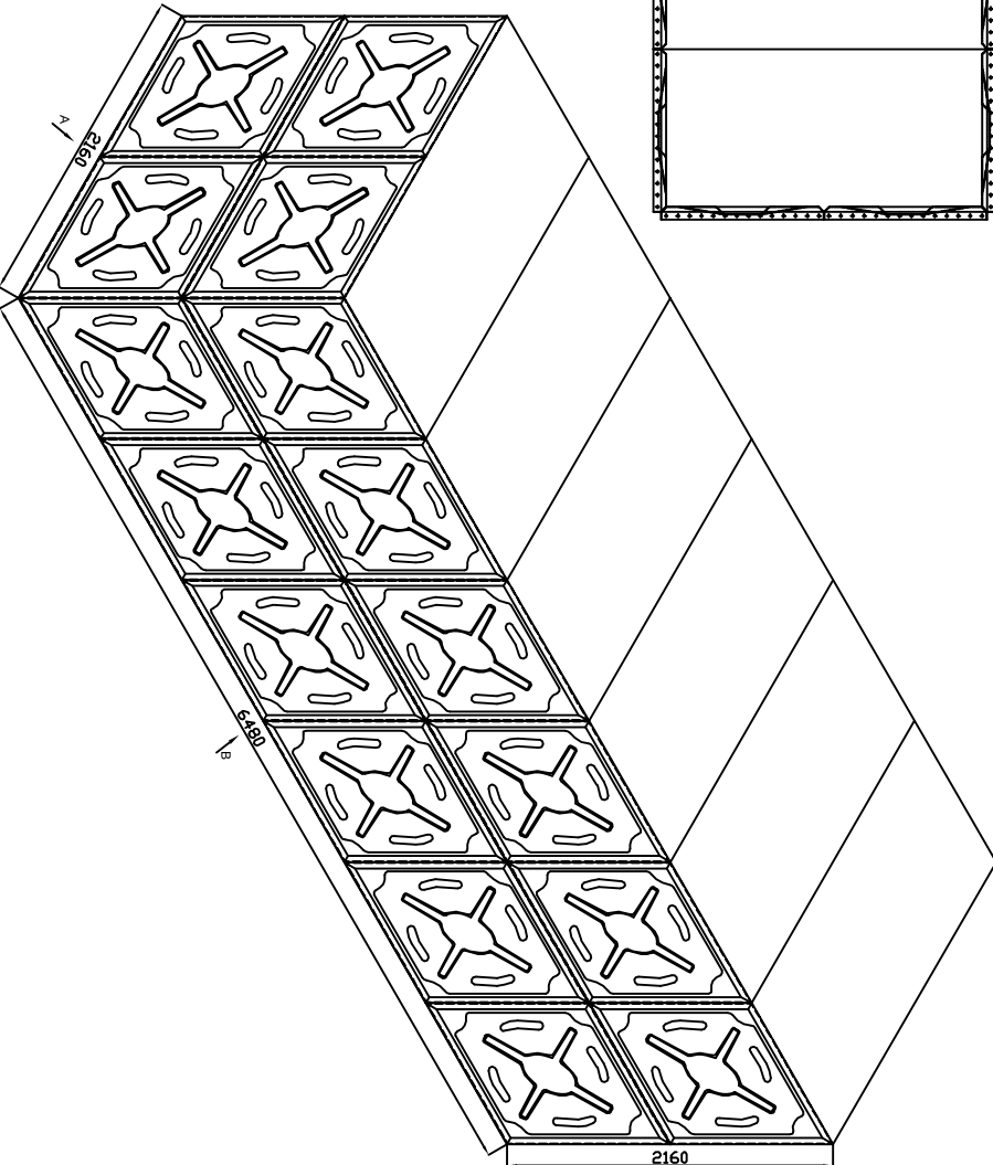
GENEL GÖRÜNÜŞÜ
