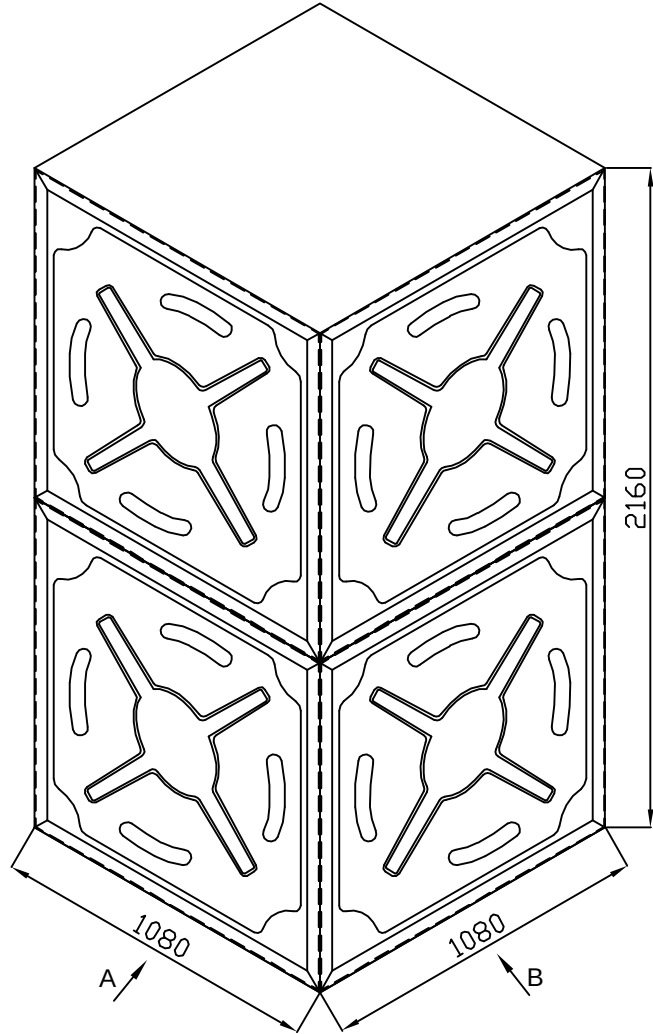
GENEL GÖRÜNÜŞ
