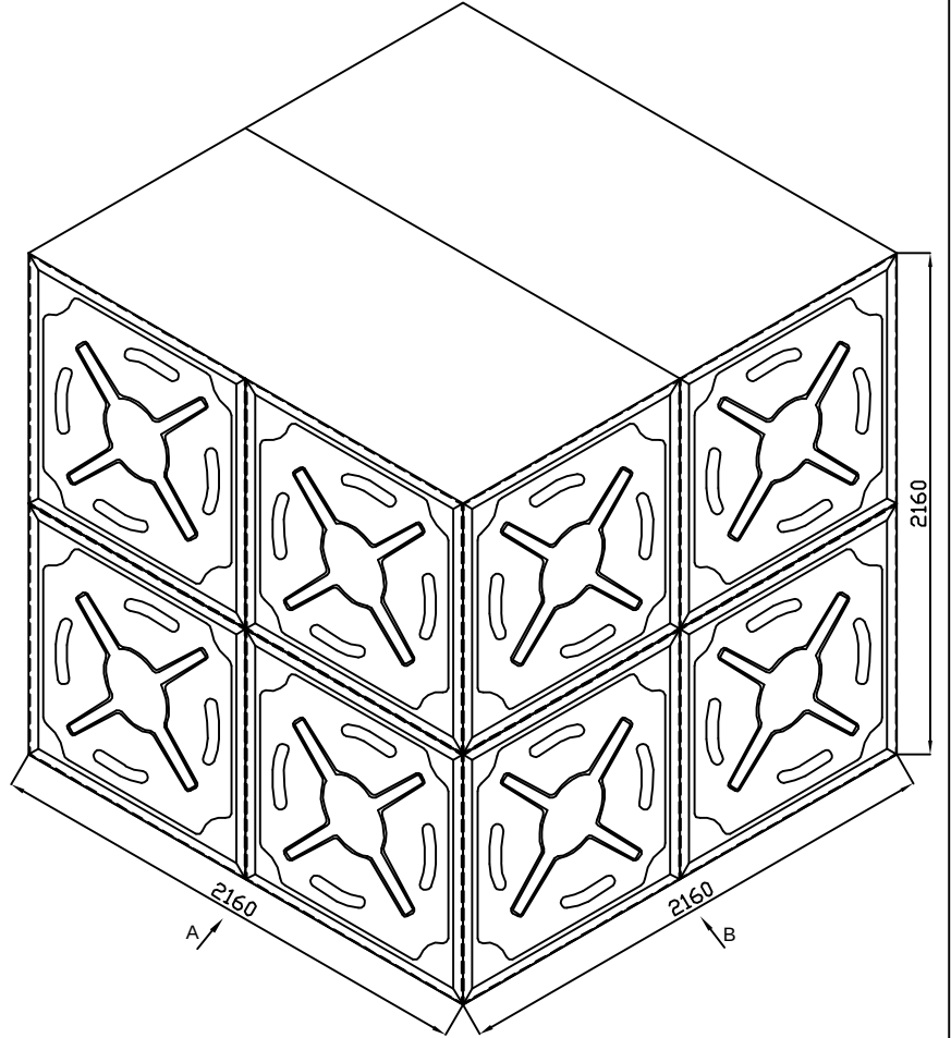
GENEL GÖRÜNÜŞÜ
