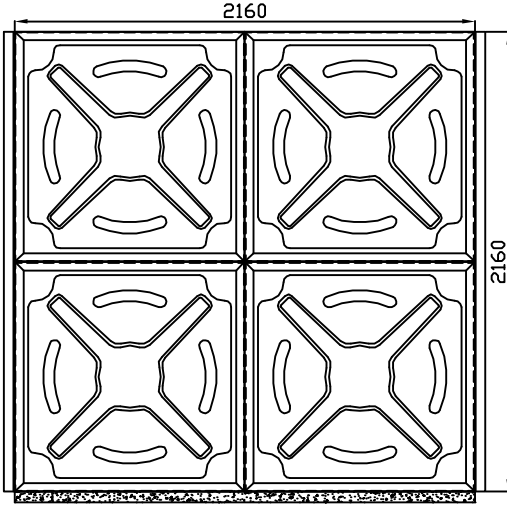
B GÖRÜNÜŞÜ
